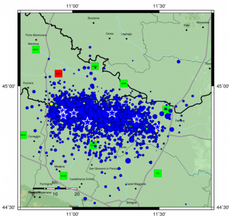
Mappa Epicentrale della Sequenza Sismica per il periodo 16-05-2012 : 03-09-2012
