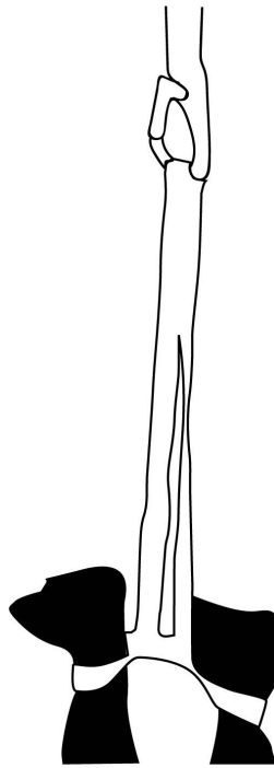
Figura 13. Cinghia di salvataggio di classe C. È progettata in modo che la persona da salvata sia mantenuta a testa in giù, con le cinghie intorno alle caviglie durante l'azione di soccorso. Se possibile, le braccia e la testa devono essere protette.
