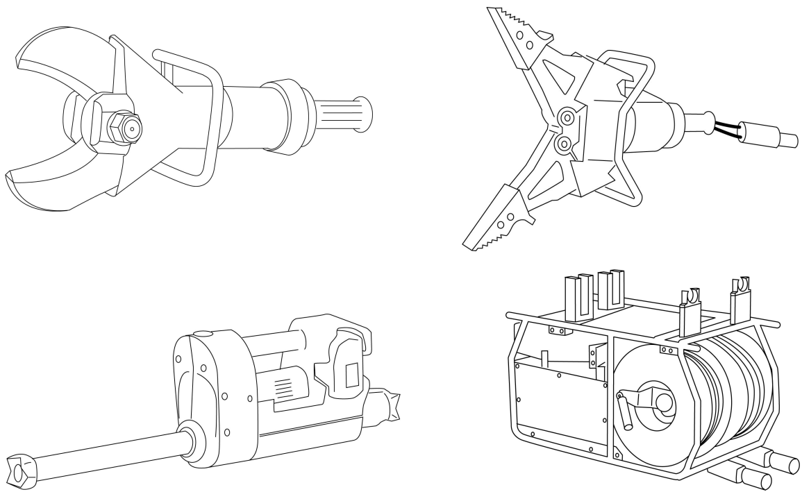
Figura 28. Esempi di dispositivi di salvataggio . In senso orario: tenaglia/trancia idraulica e a pinza; divaricatore lineare elettroidraulico; unità di potenza per il comando dotata di accorgimenti per il collegamento rapido.
