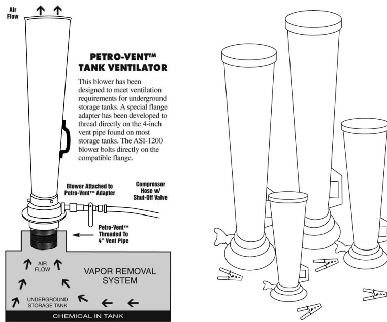
Figura 26. Eiettori ad aria compressa , pensati per ambienti particolari. Si notino nell'immagine di destra le pinze per il collegamento equipotenziale contro i fenomeni elettrostatici.
