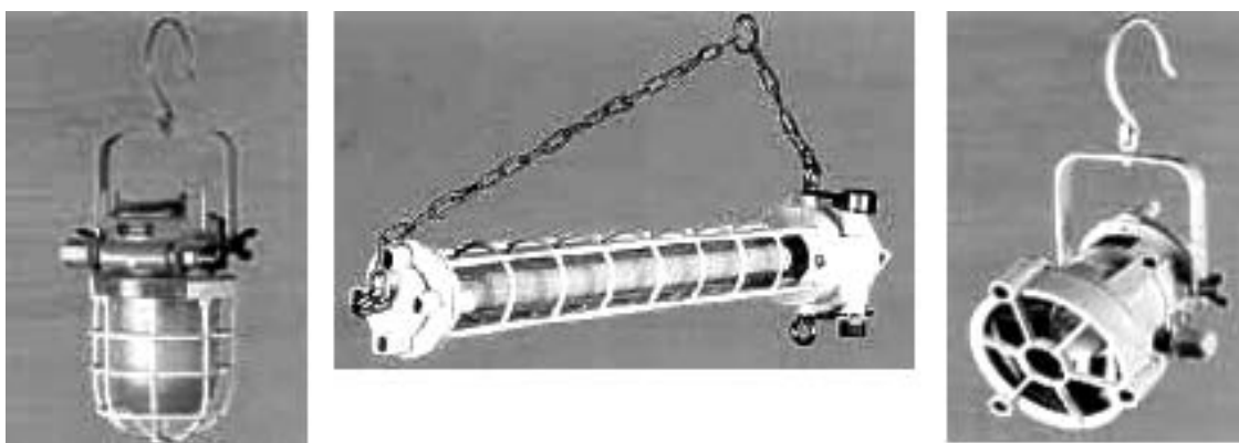
Figura 30. Esempi di lampade funzionanti ad aria compressa .
