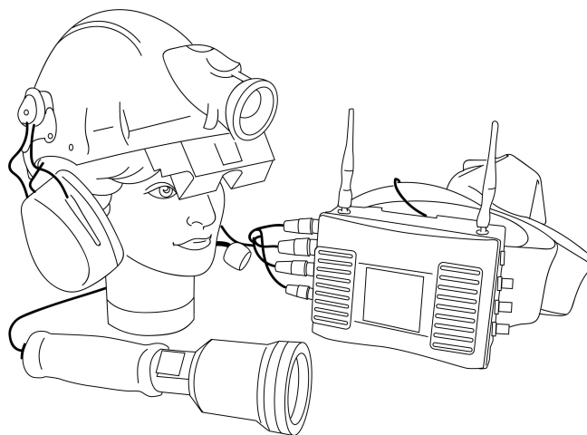
Fig. 27 Esempio di sistema di comunicazione bidirezionale audio e video che consente di tenere in contatto l'operatore all'interno dell'ambiente confinato e un operatore esterno. L'immagine mostra un sistema dotato di due sistemi di acquisizione di immagini, uno sul casco e l'altro brandeggiabile con funzioni anche di torcia. Il casco è anche dotato di un visore/schermo che permette in remoto di interagire in diretta con l'operatore. Il tutto è completato da un sistema audio di comunicazione.
