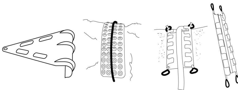
Esempi di paraspigoli
