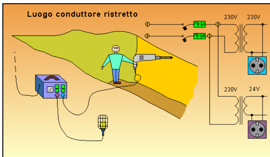
Figura 8.1 - Esempio di possibile luogo conduttore ristretto
