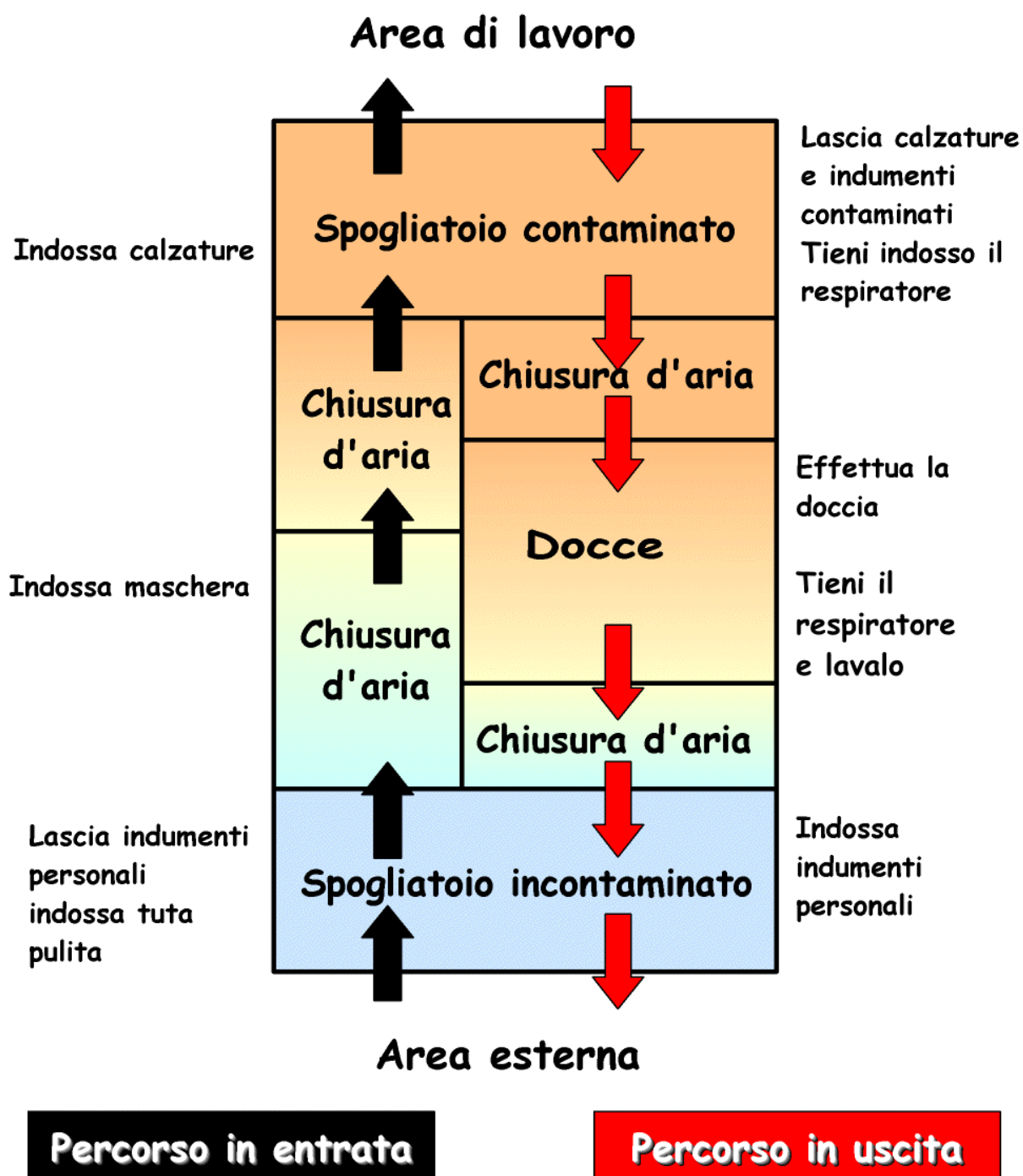
Figura 45 - Area di decontaminazione del personale
