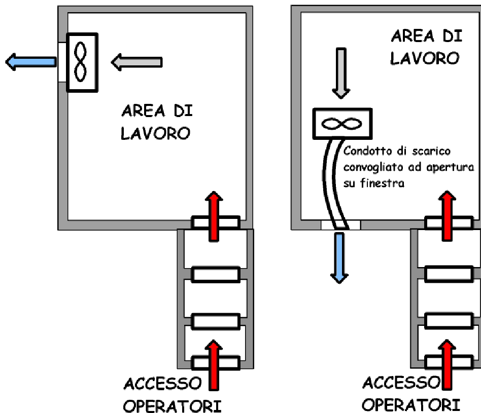
Figura 44 - Confinamento dinamico con estrattori d'aria
